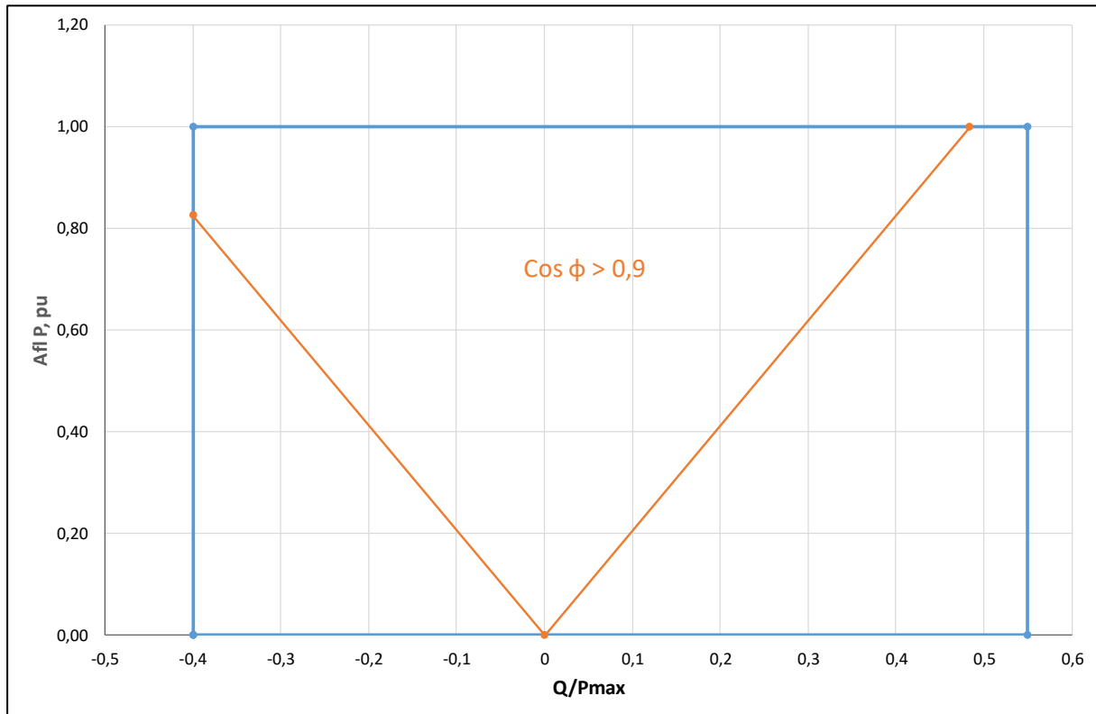
Mynd 7 P-Q/ P_{\max} svið fyrir orkulundi. Orkulundir eiga að vera færir um að vinna innan ferhyrningsins á myndinni.
