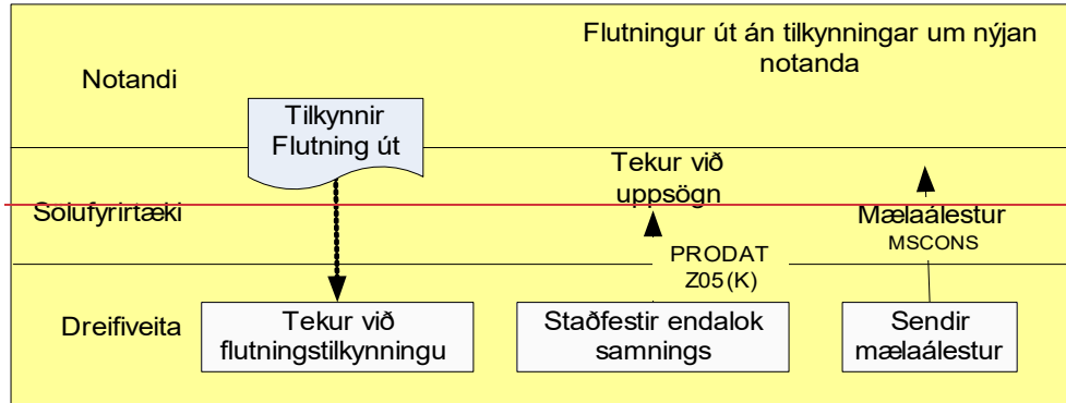
Mynd 3: Notandaskipti
